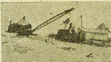
Նկ. 75. Բասկունչակ լճից մեքենաների միջոցով աղ ստանալը.
