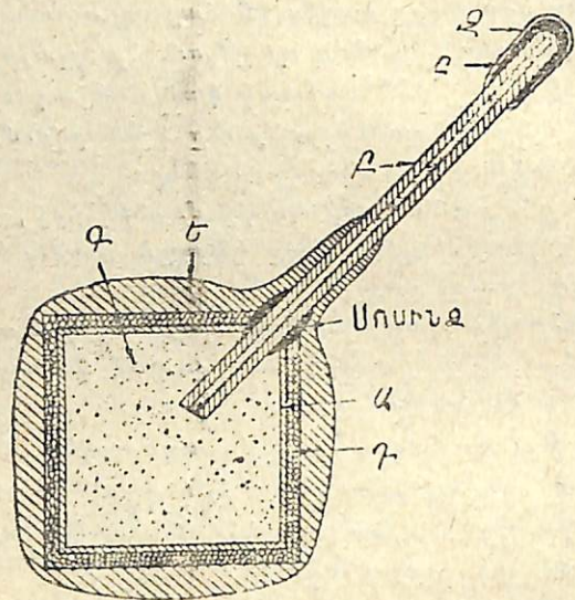
Նկ. 1 Պայթուցիկ ծրարի կտրվածքը
