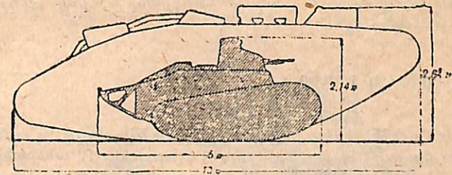
Նկ. 4 Ռենո տանկի (զնայրած է) և Ռեկարդո-յի համեմատական մեծությունը
