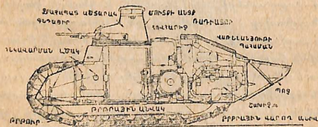
Նկ. 2 թեթև Ռենո տանկի կառվածքը
