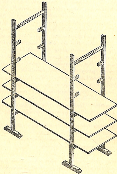
Ձեւ 12. — Վանդակ եղեգնայ վեց յարկ. երկայն, 2մ, 40. Լայն 0մ, 75:
