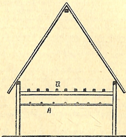
Աււ 14. — Տաղաւար շերամ բուծանելոյ, բարձր 6 մետր, լայն 4 մետր:
