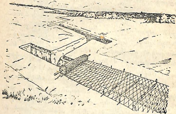
նկ. 14. Խրամուղիների ծածկույթը:
