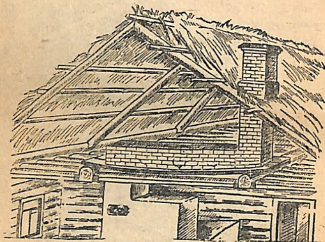
Նկ. 3. Միակ կառուցված շեղակի ծխանելույզ — բարակ տախտակների վրա, վորոնք կորացել են, վորից և վառարանը ճեղքվածքներ են տվել:
