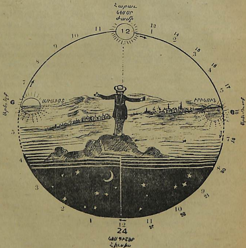
Պատ. 3. — Երկրի չորս կողմերը
