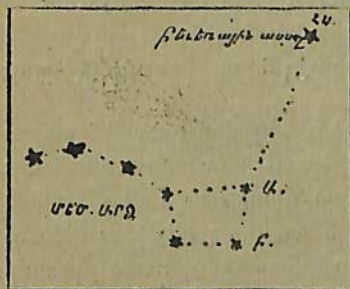
Պատ. 5. — Բեւեռային աստղ
