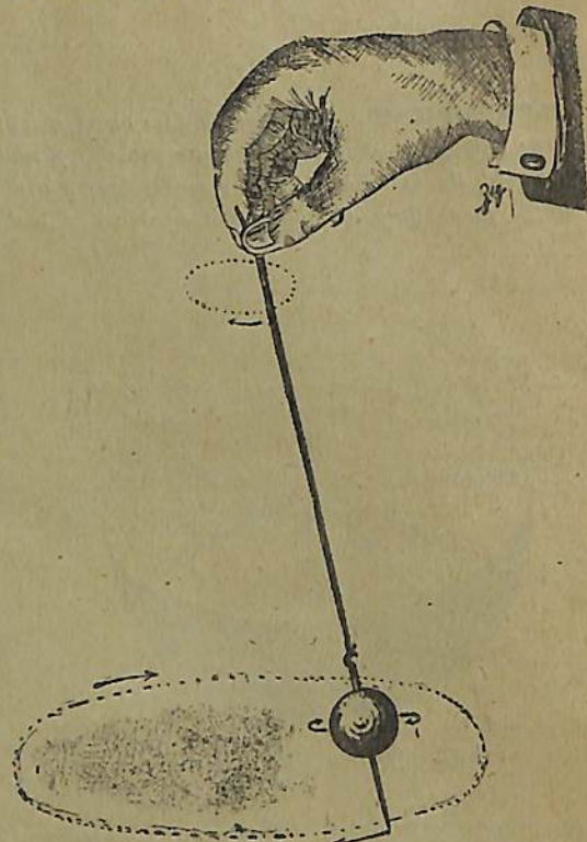
Պատ. 41. — Թաւալում եւ Տարեկան Շարժում (Հնդկական)
