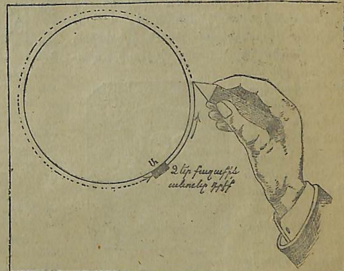
Պատ. 13. — Երկրի կտրուկները
