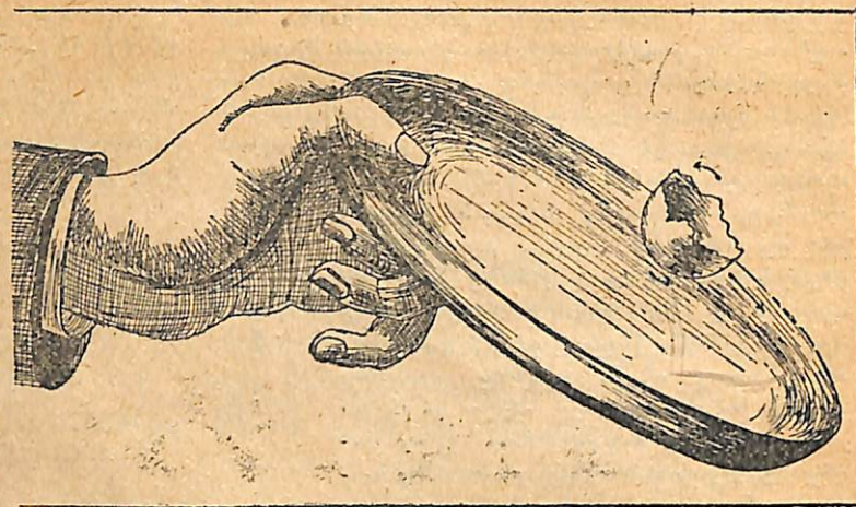
Պատ. 8. — Երկրի քաւալումը եւ տարեկան տարժումը ցուցնող փորձ
