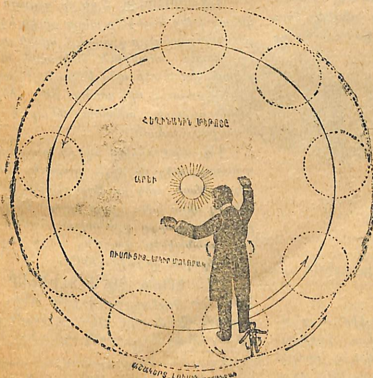
Պատ. 7. — Թաւալումի եւ տարեկան շարժումի փորձ
