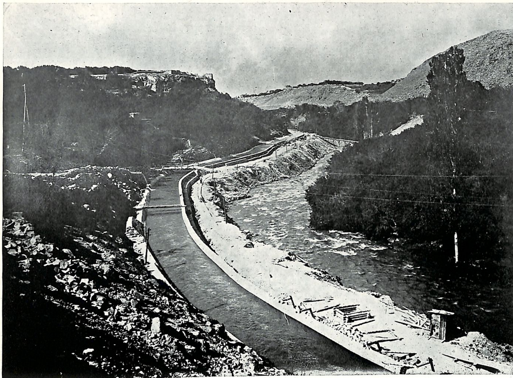
ԵՐԵՒԱՆԻ Բ. ՀԻԴՐՈԵԼԵԲՏՐԱԿԱՅԱՆԻ ԶՐԱՆՑՔԸ
