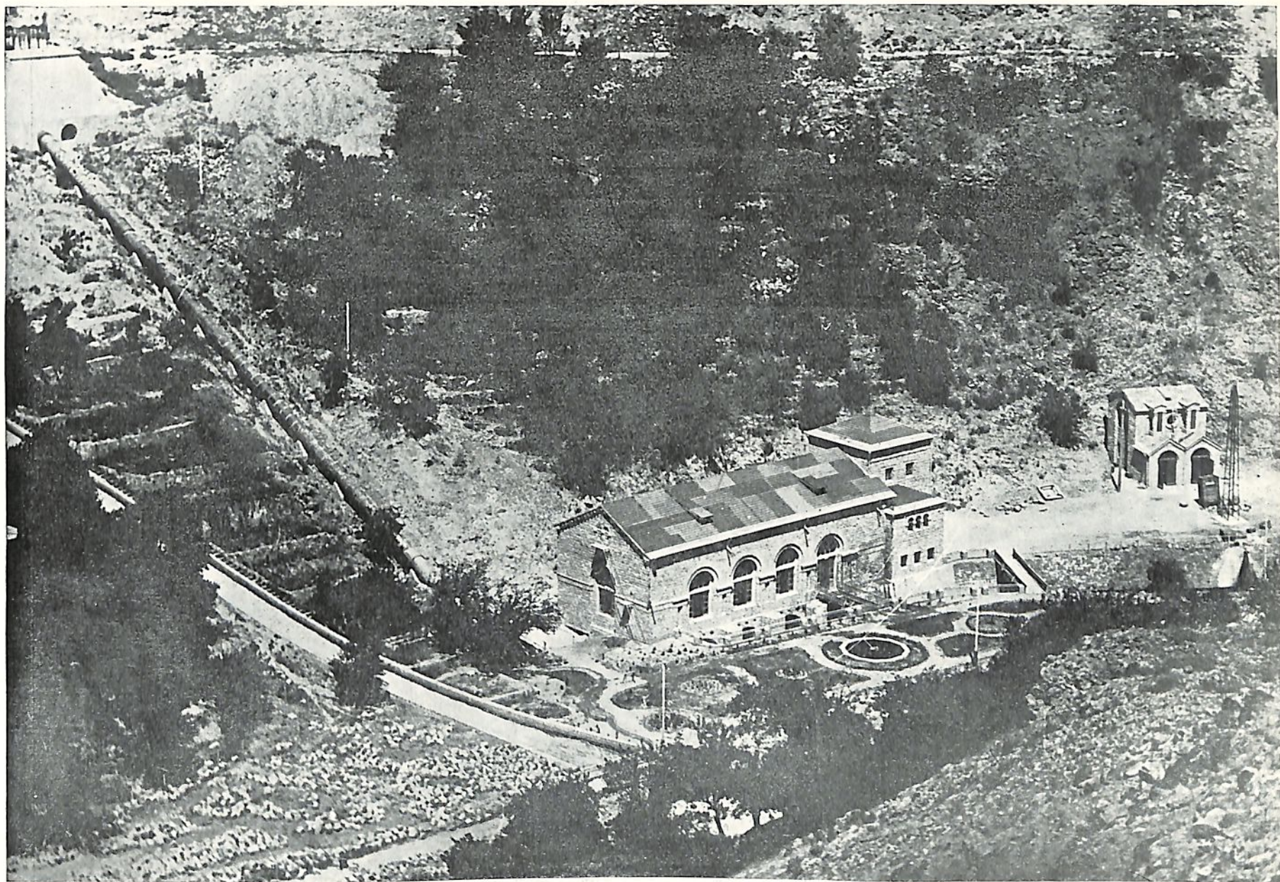
ԵՐԵՎԱՆԻ Ա. ՀԻԴՐՈԵԼԵԲՏՐԱԿԱՅԱՆԻ ԸՆԴՀԱՆՈՒՐ ՏԵՍԻՍ (ԵՐԳԵՍ)
