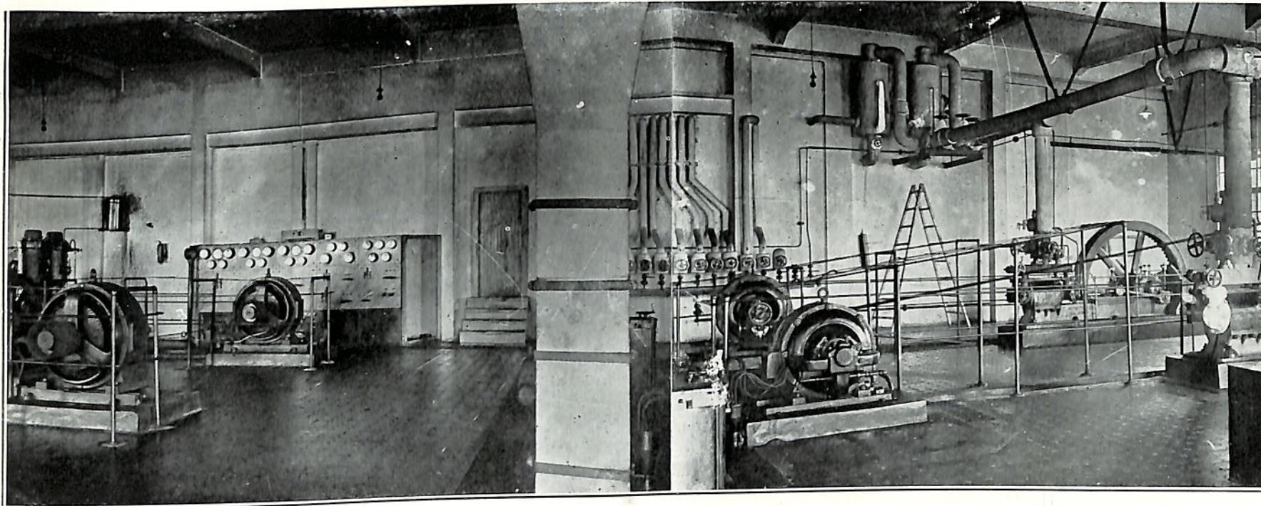
ՁԷԹԻ ԳՈՐԾԱՐԱՆԸ — ԵՐԵՒԱՆ
