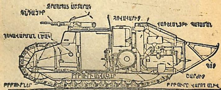
Նկ. 14. Ռենո տանկի կառվածքը
