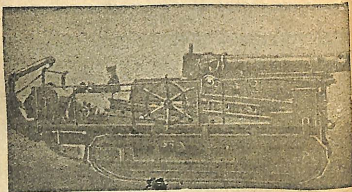
Նկ. 6. Շուգելի 240 ս. թվրապոր հորեցը յերթական դրությամբ
