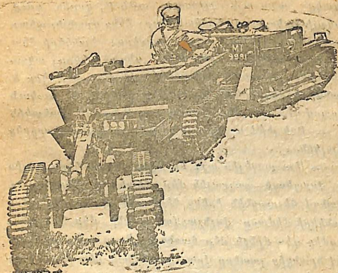
Նկ. 18. Հակա տանկային թնդանոթ մեխանիզական քարշոյ
