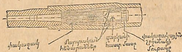
Նկ. 16. Փակադակի մարտական հենարանները փակադակը միացնում են փողատուփի հետ։
