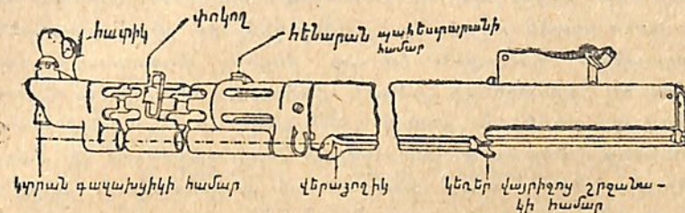
Նկ. 2. Փողատուփը և պատյանը
