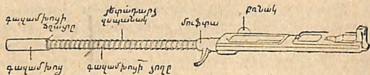
Նկ. 1 Փողը. 1—Ընդհատուն որակաձև յելուններ, 2—մուֆտա, 3—կողավոր մակերևույթ, 4—կանոնավորիչ, 5—կանոնավորիչի մանեկը, 6—փակիչի թասակը 7—փողի ավտոմատիկ փակիչը. 8—փակիչի զսպանակը, 9—բողմամբիչը, 10—կարուններ:
