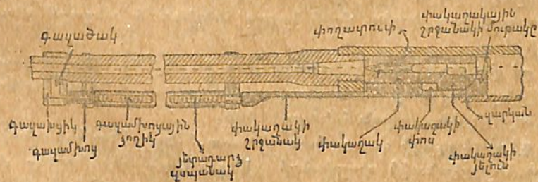
Նկ. 15. Գնդացրի մասերի ղրուկները մինչև լցնելը
