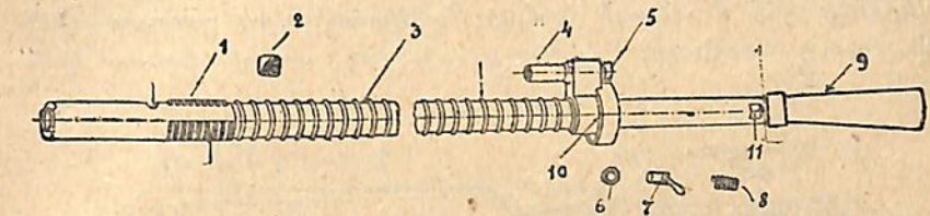
Նկ. 10. Փակադակային շրջանակը՝ զազամխոցի հետ:
