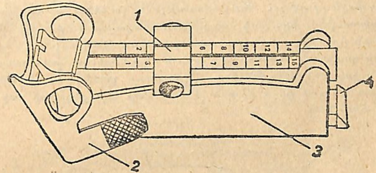
Նկ. 4. Նշանոց. 1—Անրիկ, 2—պահեստարանի մղակի յետի յեղունը նշանոցի ապահովիչով, 3—նշանոցի տուփը, 4—պահեստարանի մղակը:
