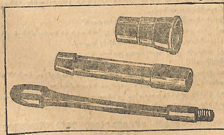
Նկ. 28. Պարկուճի հանիչը, քանդած
