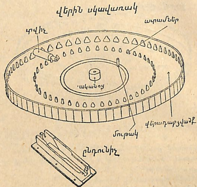
Նկ. 13 բ. Պահեստարան
