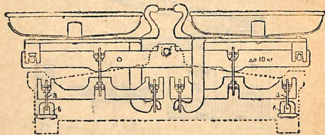
Ձեկ 5 Սեղանի կշեռք
