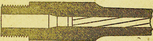
Նկ 1 Փողի ու փամփշտանոցի կտրվածքը տոլթյուն ունենալ փողաբերանի հետ, հրացա-
