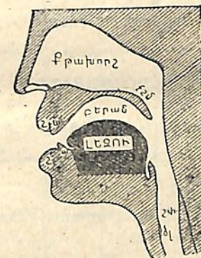
ՀՀ—շրթունք, ՀԿ—շնչափող, աա—ատամներ, քք—քիմքի շարժական մաս, ճճ—ձայնալարեր:
