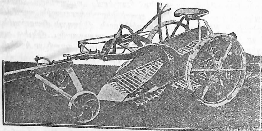
Պատկեր 11. — Գեհնապիսակի ֆաղին համար գործածուող փաթաթեա ֆաղող մեքենան :
