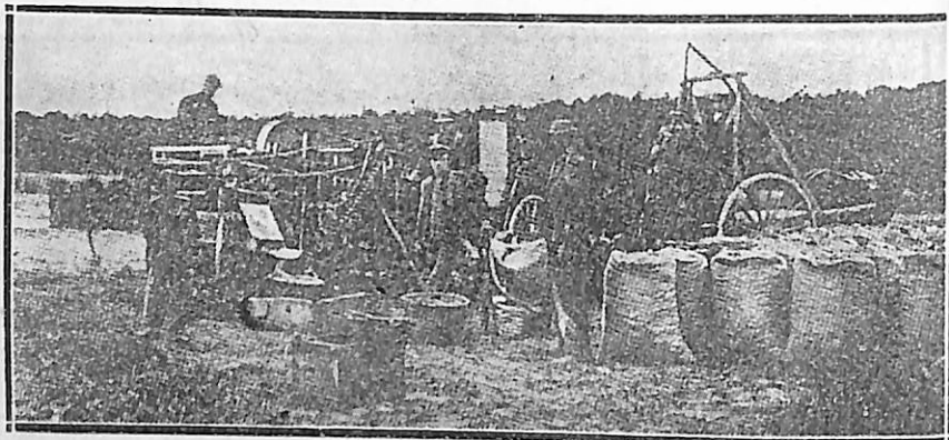
Պատկեր 17. — Գետնապիտտակ հաւաքող մեքենայ :
