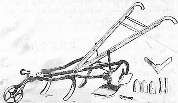
Պատկեր 4. — Միաձի մարկեղի մեքենայ
