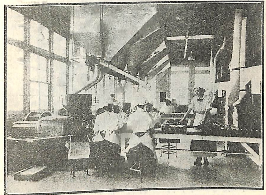
Պատկեր 28. — Գետնապիտտակի կարագի գործարանի մը աղացումի և Եիշերը լեցնելու յատուկ մեխանիզմներ։
