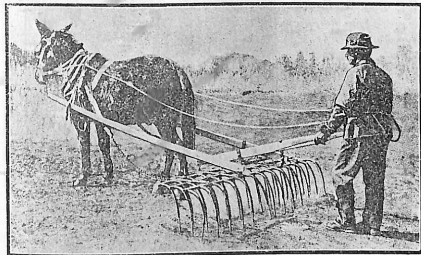
Պատկեր 5. — Վնասակար խոտերու խիլէ մեքենայ մը, որ գետնապիտտակի առաջին մարկեղման ատեն կը գործածուի:
