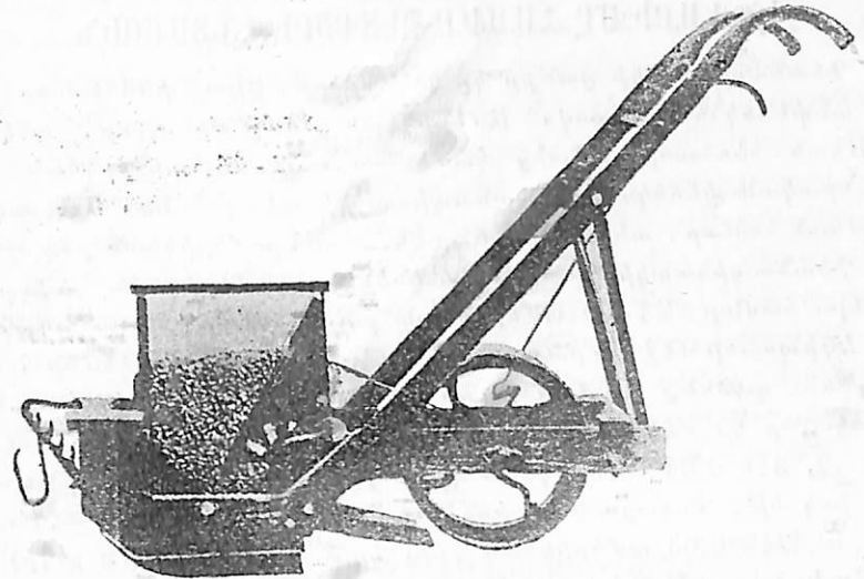
Պատկեր. 3. — Միաձի գետնապիստակի սերմնացան մեքենայ:
