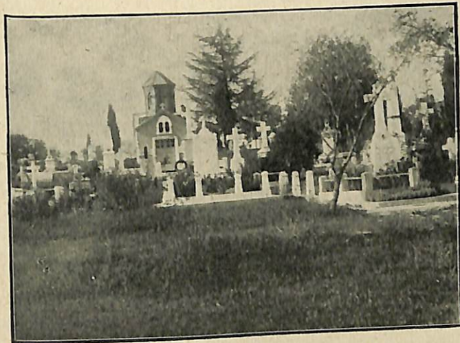
Ընդհանուր տեսարան հարաւ. կողմանէ. Ս. Սահակ ճամբուն վրայէն: Տաճարն է Մարիկեան Ընտանիք:
