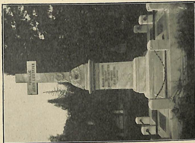
Famille Jean Loutfyan. Գերդաստան Յովհաննէս Լութֆիան:
