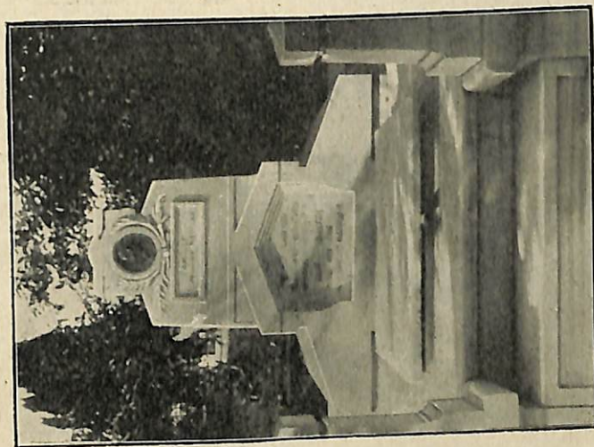
Famille Gregoire Nartian.
