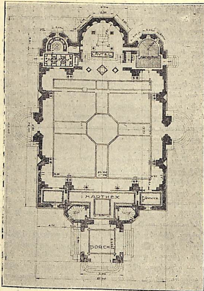
(քիւ 32) Յասակագիծ Ս. Գրիգոր Լուսաւորիչ եկեղեցւոյ
