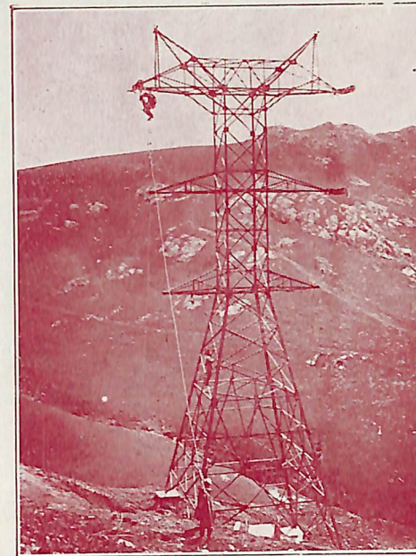
Հաղորդման գծի լարերի մոնտաժը:
