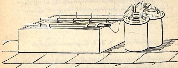
Կալուանսաձուլման արկղ:
