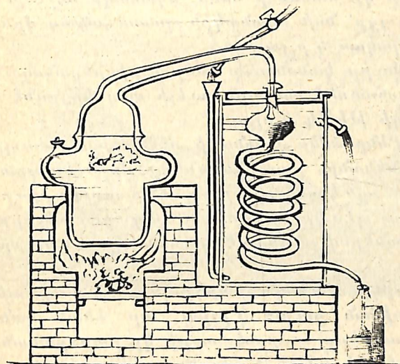
Թորեցուցիչ գործի:
