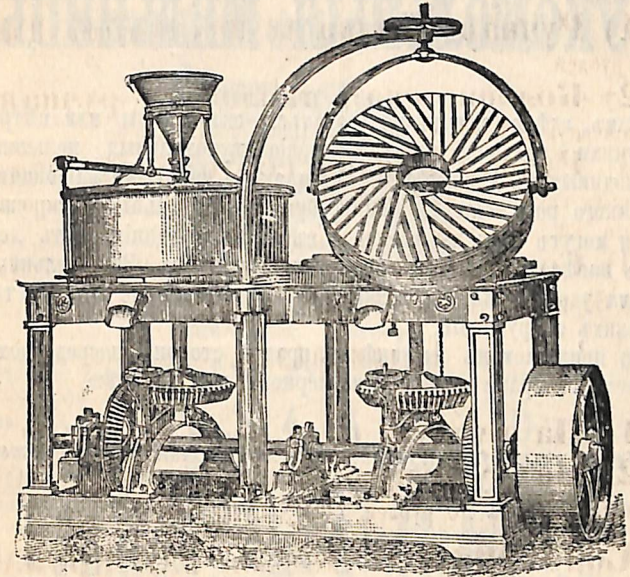
Мукомольная мельница. U. 10112
